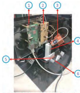
1.樹莓派 2.電壓電路 3.電磁閥 4.比色皿 5.LED燈 6.攝影機
