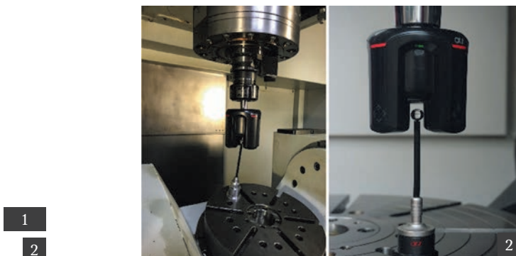
1. Alpha One 元件圖 (左：標準玻璃球棒；右：感測模組) 2. Alpha One 實際量測情形
