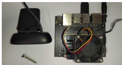
使用 Jetson Nano 之硬體架構
