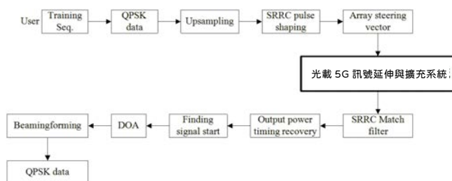
基於光載 5G 訊號之測試架構
