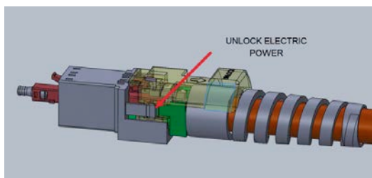
「插入即上鎖」鎖扣示意
