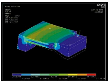
有限元素模擬機構受力狀況
