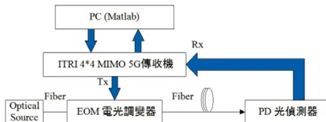
基於光載 5G 訊號之測試硬體架構
