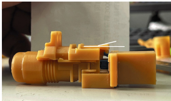
3D 列印作機構作動的驗證
