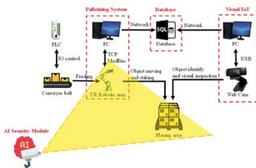
硬體架構圖
